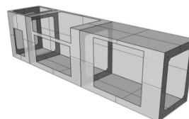
Schritt 3 Sägen der Ausschnitte für Ihre Einbaukomponenten
