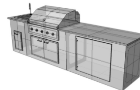
Schritt 4 Installation der Einbauteile und Montage der Arbeitsplatte
